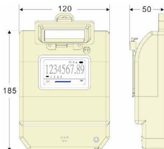
外觀尺寸 單位：mm
