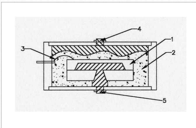
■ 壓力感應單元結構示意圖
